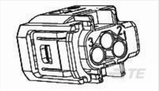
TE 产品编号1376235-1 MOS SOCKET HSG 3P ASSY
