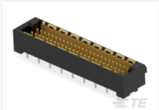
TE 产品编号354182-E MSPEED 50 M SMDTHR M1 B AB VV 137 094 *
