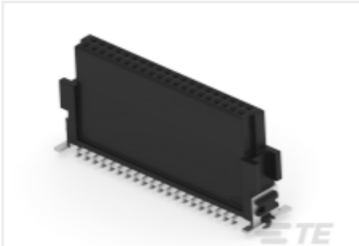
TE 产品编号354073-E SMCB 40 F AB VV 7-23 CL * H007 137 E002
