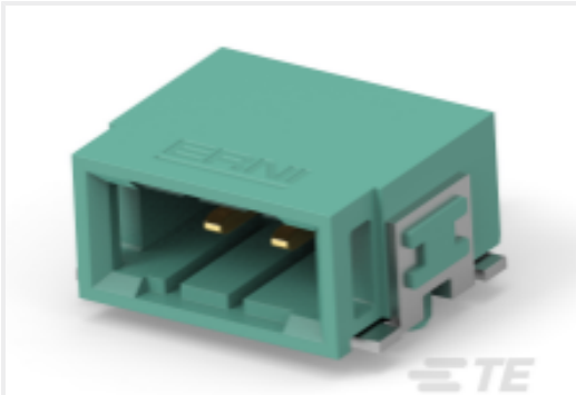
TE 产品编号234834-E SRCA 2,54 2 M 1 SMD 137 E1 167 * GURT *
