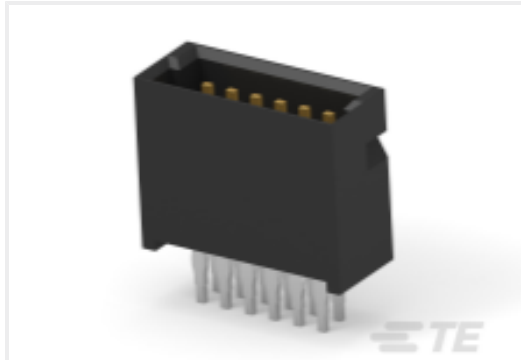
TE 产品编号064002-E SMCQ 12 M AB VV 3-04 * 2,8 0003 137 E001
