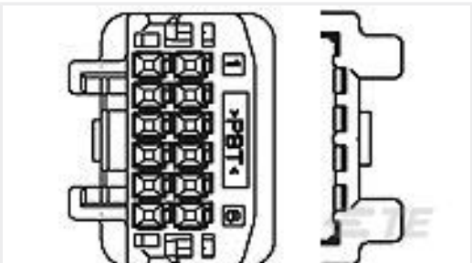
TE 产品编号170012-2 SHUR PLUG REC 20-16 MM2 0.32 X 13.97 BR
