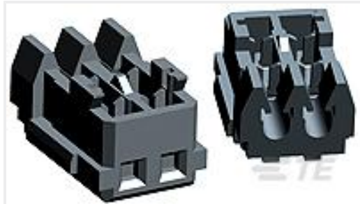
TE 产品编号353293-3 MINI CT MT REC ASSY 3P GRAY
