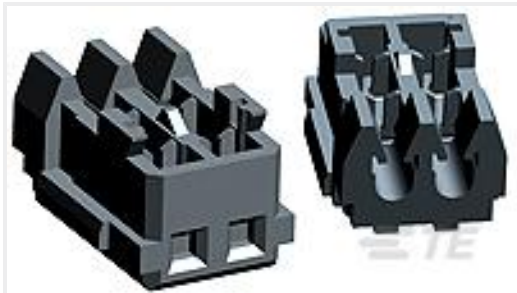
TE 产品编号353293-9 MINI CT MT REC ASSY 9P GRAY
