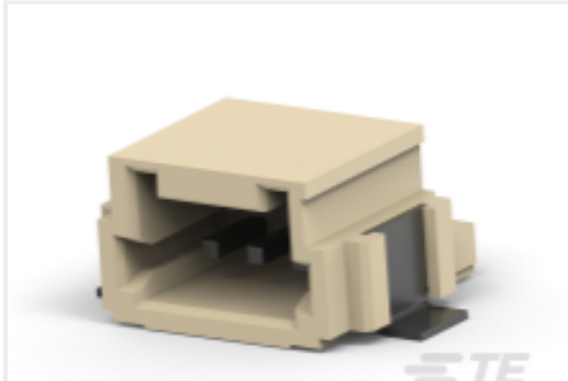
TE 产品编号 292228-3 1.5 MINI CT SGL H SMT W/O BOSS
