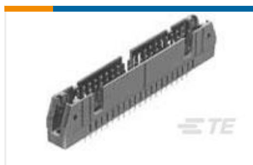
TE 产品编号 1658694-7 A/L UNIV HDR 14P ACT PIN
