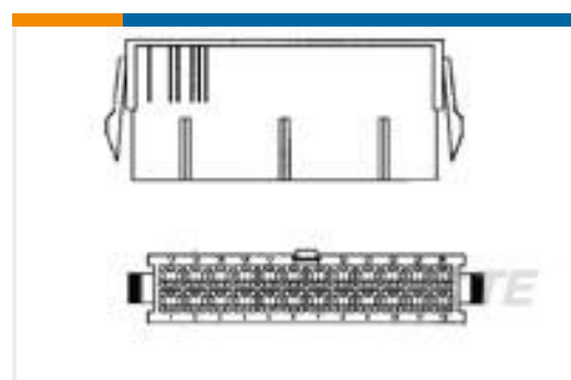
TE 产品编号2029088-4 4P PLUG VAL-U-LOK V2 PM BLK
