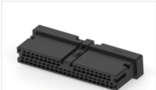
TE 产品编号4-2834461-0 MINI DYNAMIC REC HSG ASSY 40P X-KEY BLK
