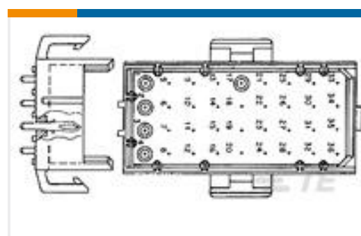
TE 产品编号2-640500-4 06P MR HDR ASSY VO LF
