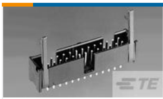
TE 产品编号1761609-3 IDC LOW PRO HDR 10P RA SHT LAT
