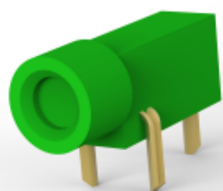
TE 产品编号 350180-5 TEST PROBE REC130 SPCL GRN GPBR
