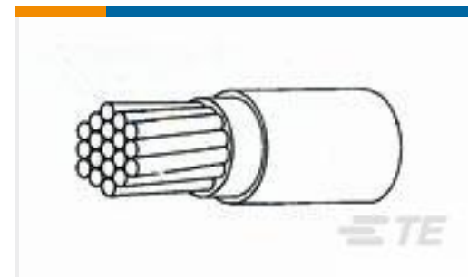
TE 产品编号2839093001 44A0211-14-2
