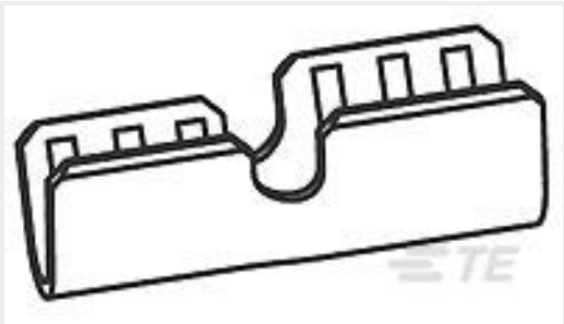
TE 产品编号61021-1 SPLICE 18-16 AWG .0126 NPST
