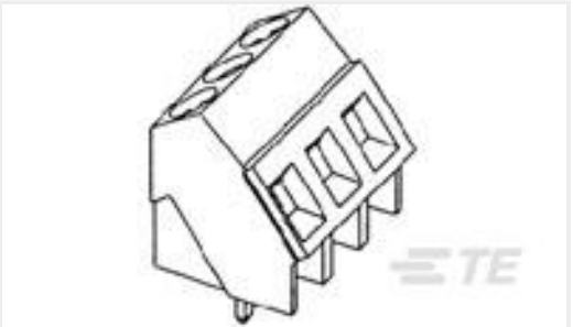
TE 产品编号1546074-2 2 POS 5.08MM TERMI-BLOK TOP WI
