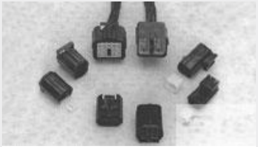
TE 产品编号344263-1 13 WAY REC HSG. SIL. SEALECONO
