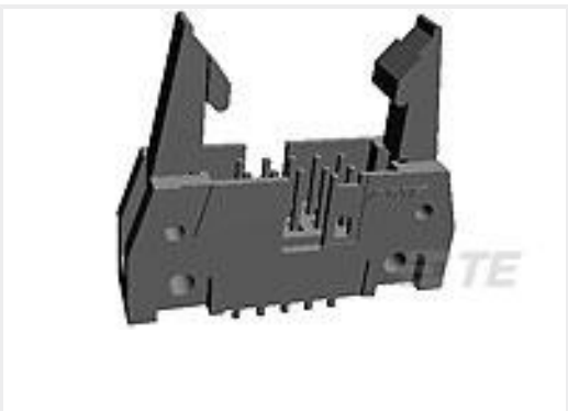
TE 产品编号2-5499206-1 A/L UNIV HDR 10P VERT LAT B
