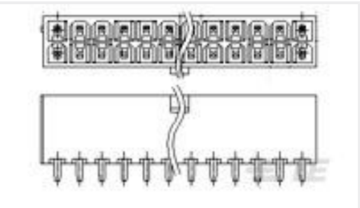
TE 产品编号4-1775099-6 ATX PWR CONN 18 POS
