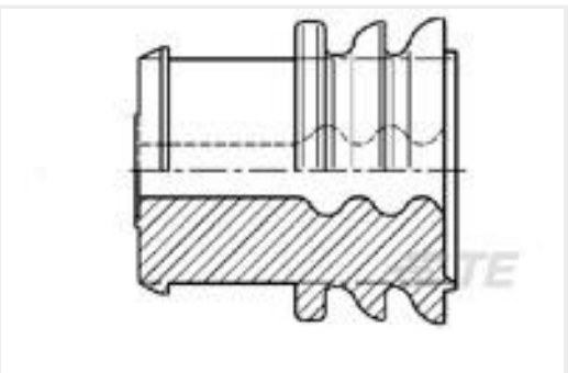
TE 产品编号963243-1 EINZELDRAHTDICHTUNG
