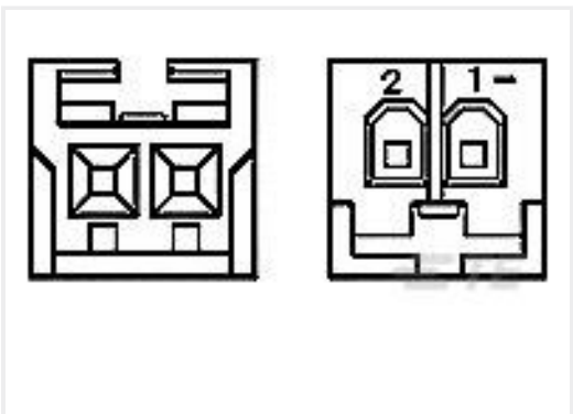
TE 产品编号172486-3 3P REC HSG CRIMP EI SER
