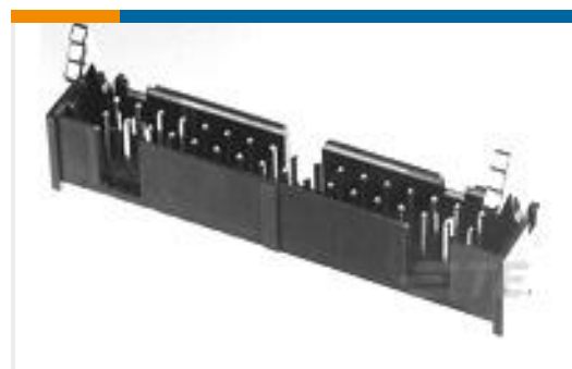
TE 产品编号1-1761606-1 IDC LOW PRO HDR 34P VERT LG LAT BLK
