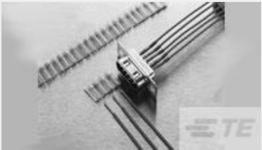
TE 产品编号626152-000 D-704-0043
