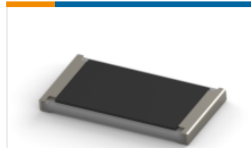
TE 产品编号3-2176070-3 SMD 功率电阻器：2 瓦特，3521 系列
