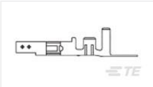
TE 产品编号1586317-3 VAL-U-LOK SKT PHBZ SN 26-22 LP
