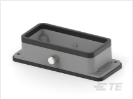
TE 产品编号T1550160000-001 H16B-AG-RC
