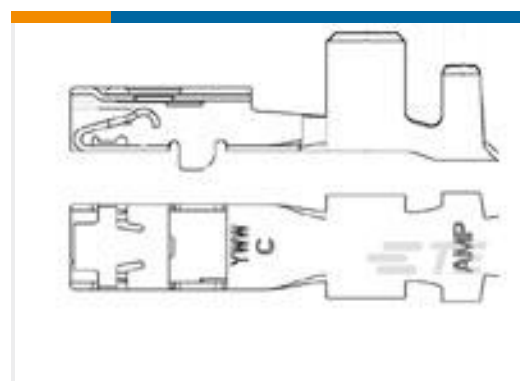
TE 产品编号1326030-6 2.8MM RECPL,UNSEAL,18-20,REVREE
