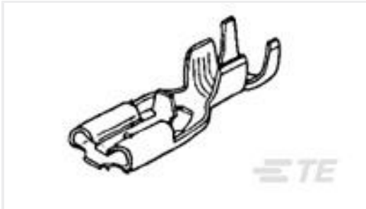
TE 产品编号170326-1 187 PL MKII REC. 18-14AWG PTBR
