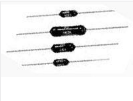
TE 产品编号6-1879672-7 H8 48R7 0.1% 25PPM
