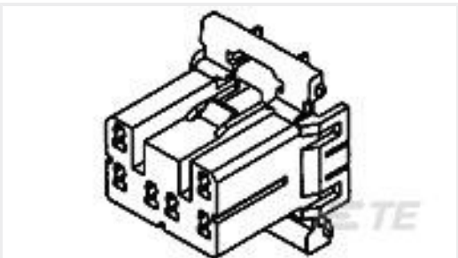
TE 产品编号173853-1 070 MULTILOCK PLUG 18P
