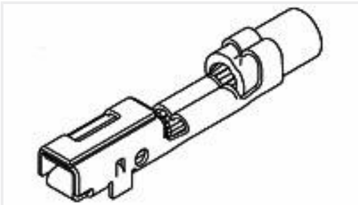
TE 产品编号368084-1 090III NON SLD REC(SQ0.85-1.25)
