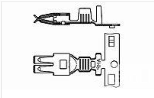
TE 产品编号963893-1 RECEPTACLE CONTACT 6,3
