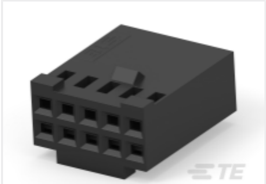
TE 产品编号 87631-5 10 MODIV HSG COMP DR .100 POL
