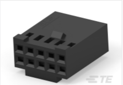
TE 产品编号 87631-6 10 MODIV HSG DR MRKD .100 POL
