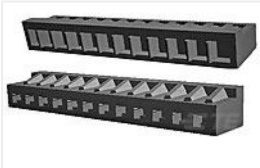
TE 产品编号172890-8 8P 2MM MINI AMP-IN HDR HSG
