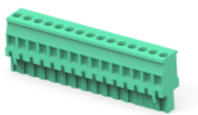
TE 产品编号 3-284047-9 TERMI-BLOK VERTICAL PLUG STACK
