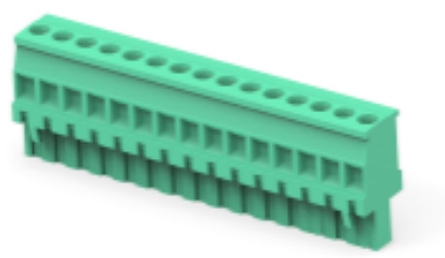
TE 产品编号 3-284047-8 TERMI-BLOK VERTICAL PLUG STACK
