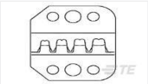
TE 产品编号217212-2 PRO-CR DIE, CES
