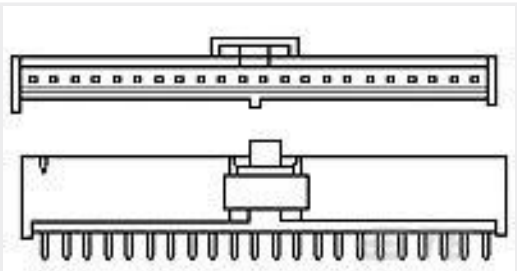
TE 产品编号3-100669-1 Z-PACK M.CONN.175P.
