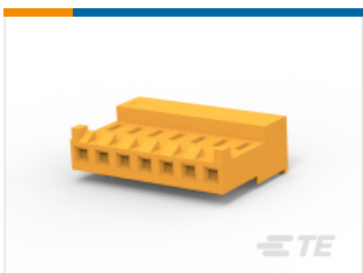
TE 产品编号 3-644878-7 07P MTA156 ASSY ON TAPE LF
