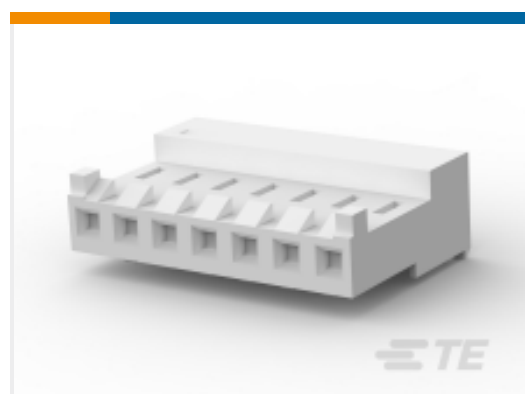
TE 产品编号 3-643820-7 07P MTA156 CONN ASSY 24AWG LF
