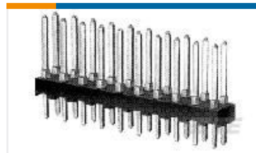
TE 产品编号1-87227-0 20 MODII HDR DRST UNSHRD .100
