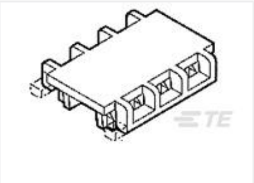
TE 产品编号1-643071-4 14P MTA156 FD-THRU COVER
