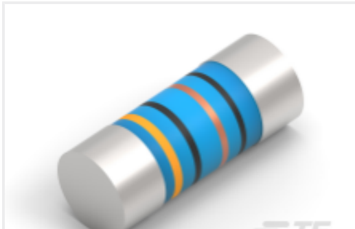
TE 产品编号8-2176316-5 MELF SMA-A 47R 1% 50PPM 0207 1W
