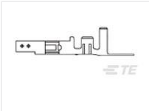
TE 产品编号794958-3 VAL-U-LOK SKT PHBZ SN 22-26AWG
