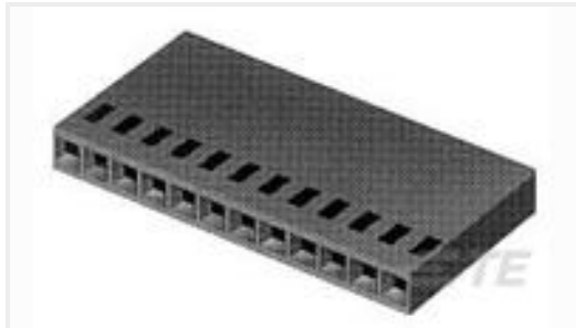
TE 产品编号7-87499-2 01 MODIV HSG COMP SR .100CL
