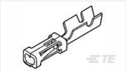
TE 产品编号5-103171-4 MOD IV RECP PLTD 30 DPLX LF
