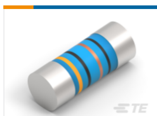
TE 产品编号3-2176315-3 MELF SMA_A 47K 0.1% 15PPM 0204 0.4W
