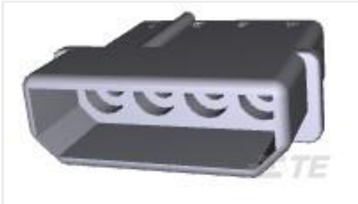
TE 产品编号1-480426-0 04P CMNL CAP HSG F/H NATL
