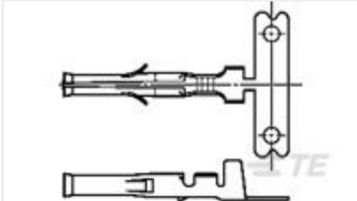
TE 产品编号350628-5 .062 COMM P&S SOK AUNI/BR
