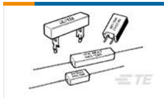
TE 产品编号1-1623795-2 SQP10 47R 5% WIRE
