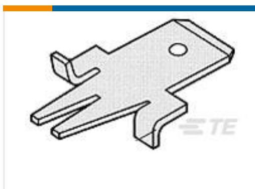
TE 产品编号63067-1 250 FASTON TAB TPBR
